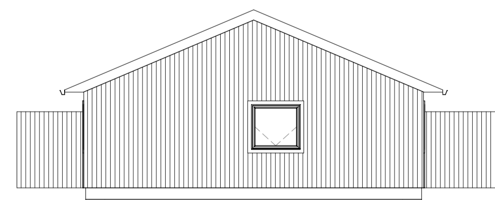
3 ÚTLIT 2 1 : 100
