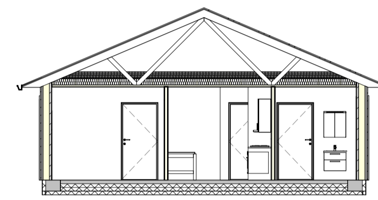
6 ÞVERNSÍÐ 1 : 100
