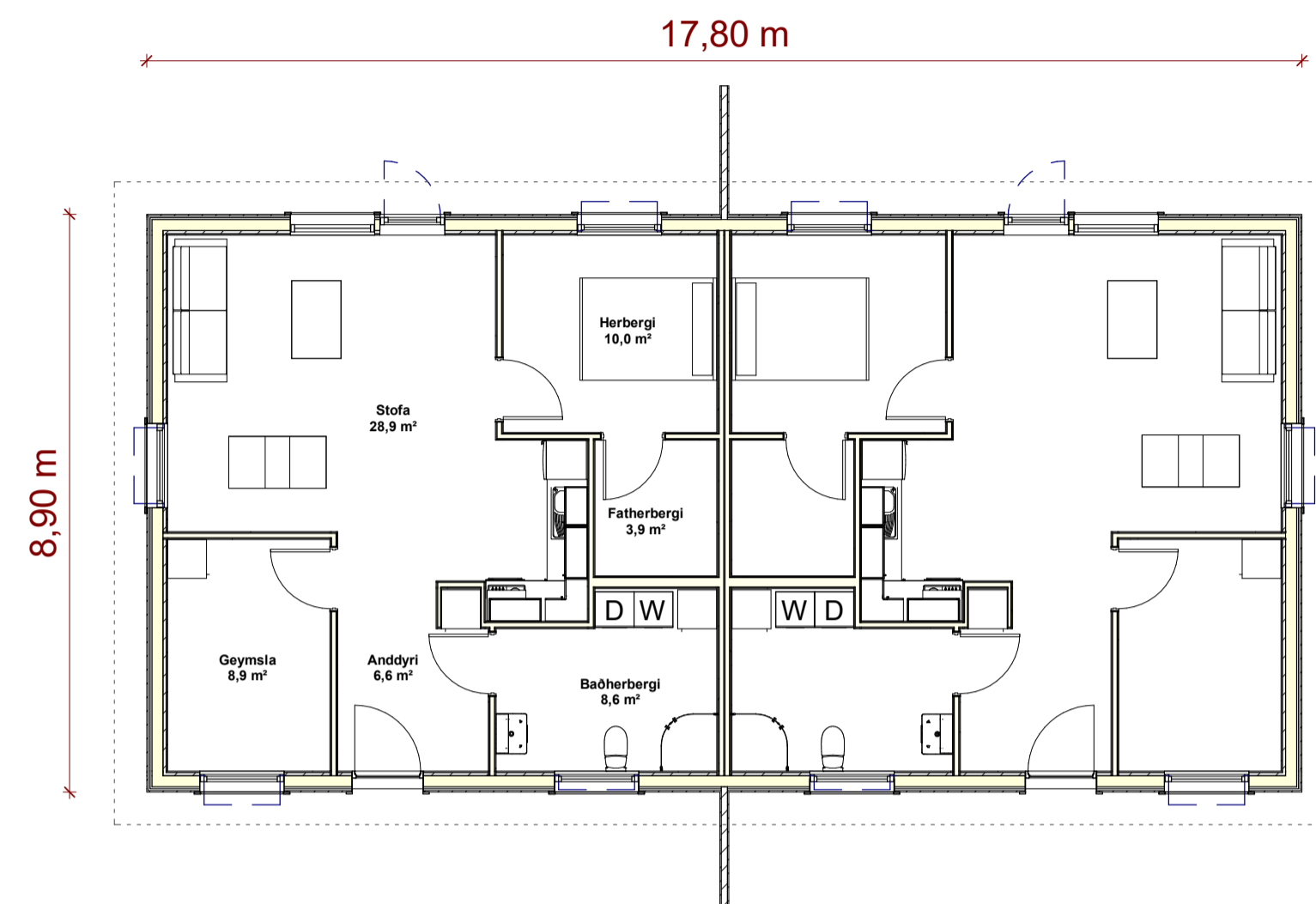
1 GRUNNMYND 1 : 100
