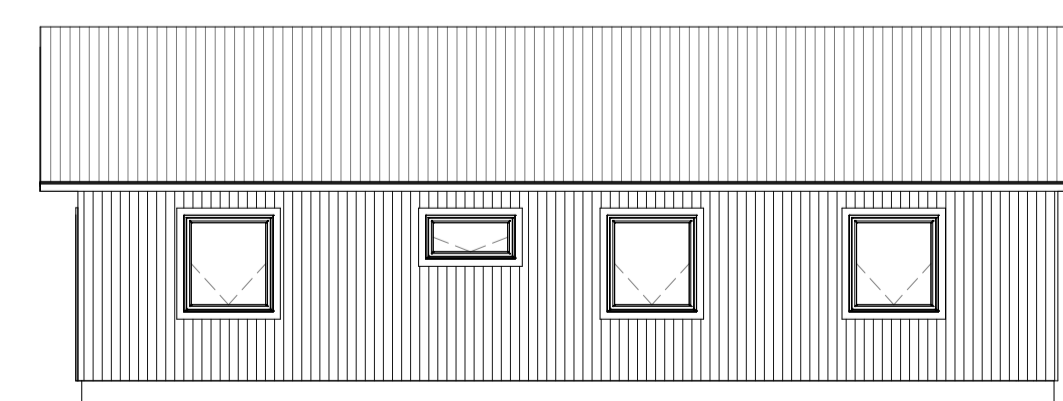
5 ÚTLIT 4 1 : 100
