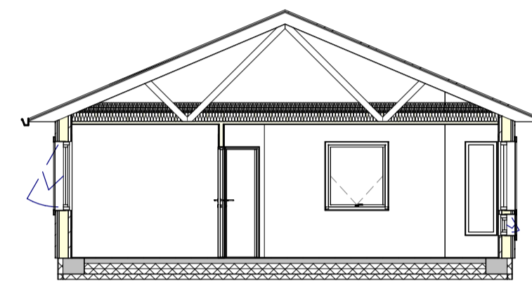
6 ÞVERNID 1 : 100
