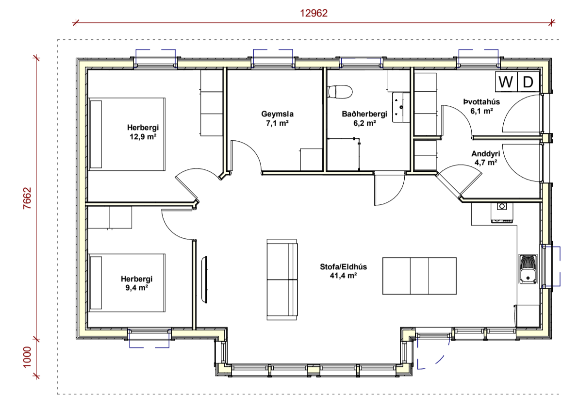
1 GRUNNMYND 1 : 100
