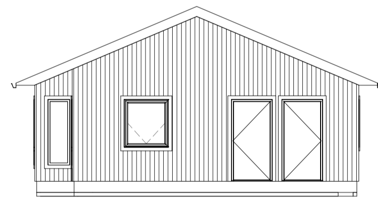
3 ÚTLIT 2 1 : 100
