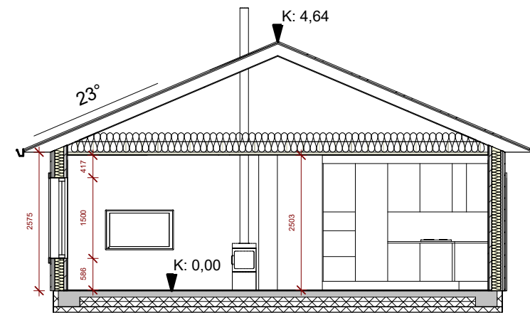
5 Þversnið 1 : 100
