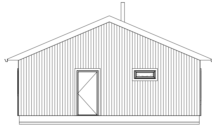
1 Útlit A 1 : 100
