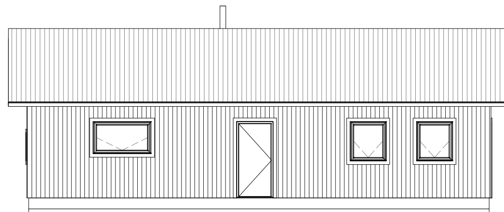
2 Útlit B 1 : 100
