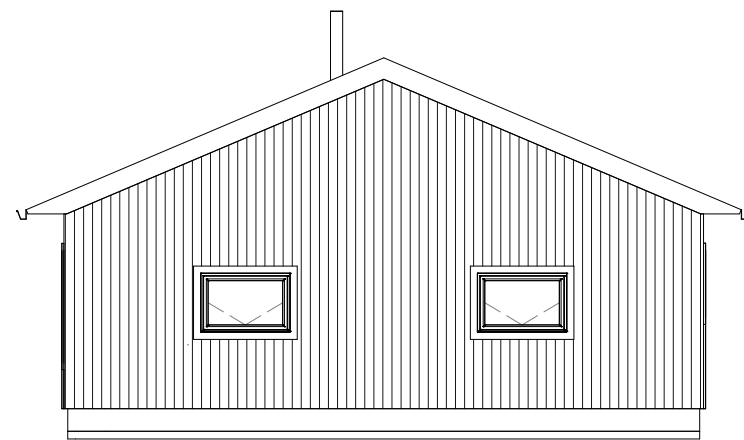
3 Útlit C 1 : 100
