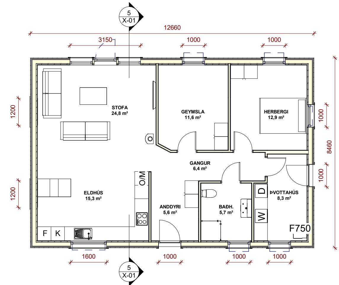
6 GRUNNMYND 1 : 100
