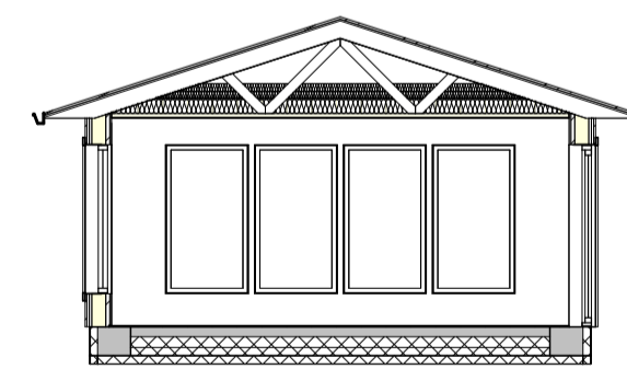
6 ÞVERSNIÐ 1 : 100
