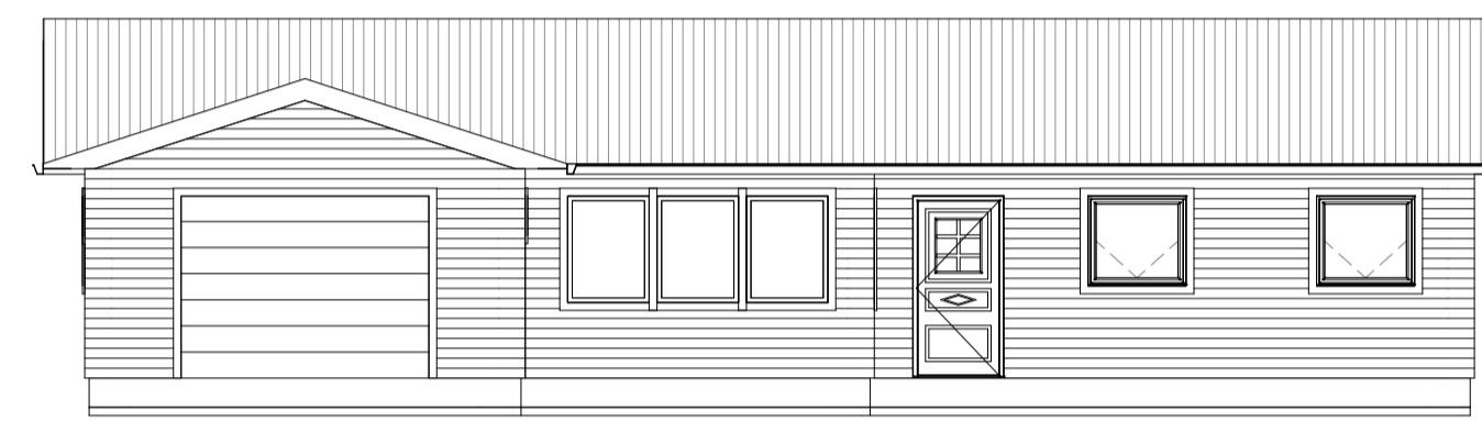
3 ÚTLIT 3 1 : 100
