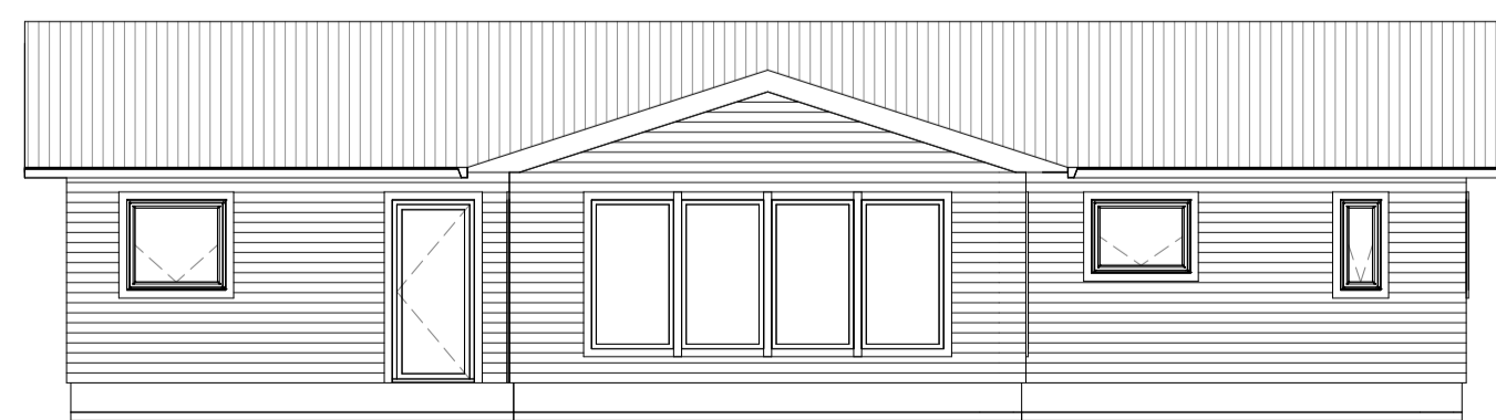
2 ÚTLIT 2 1 : 100
