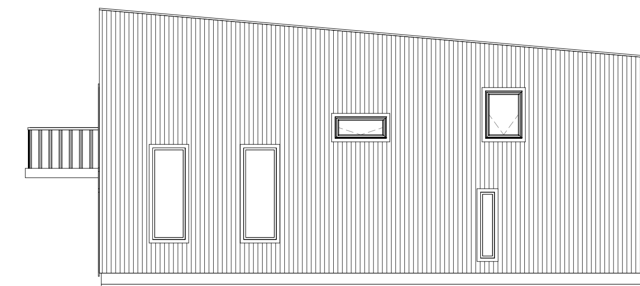
5 ÚTLIT 2 1 : 100
