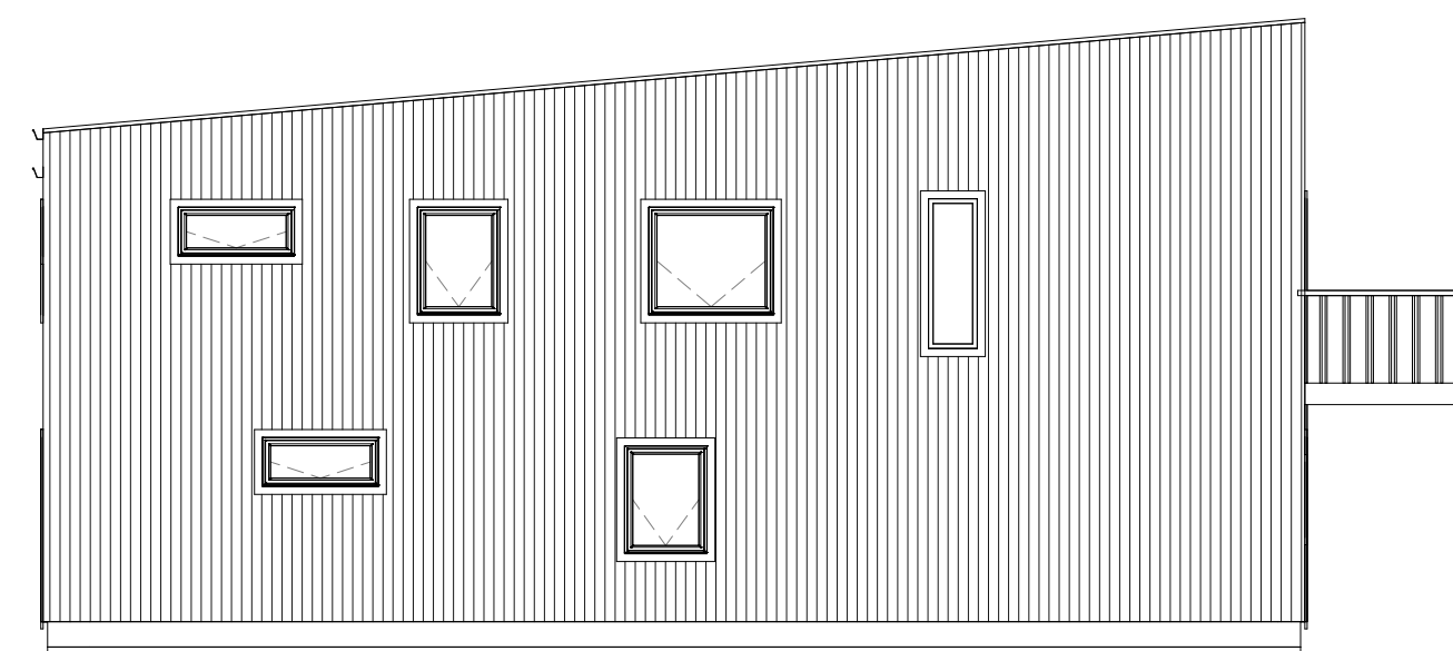
6 ÚTLIT 3 1 : 100
