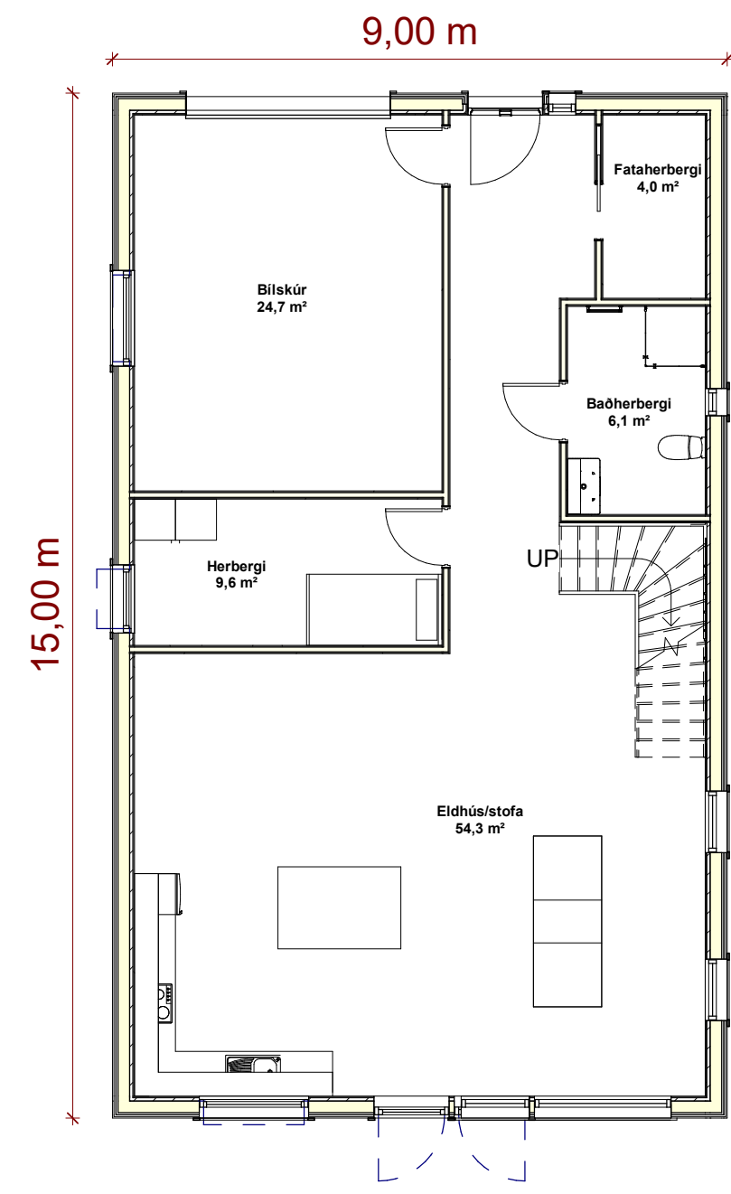
2 GRUNNMYND 1 : 100
