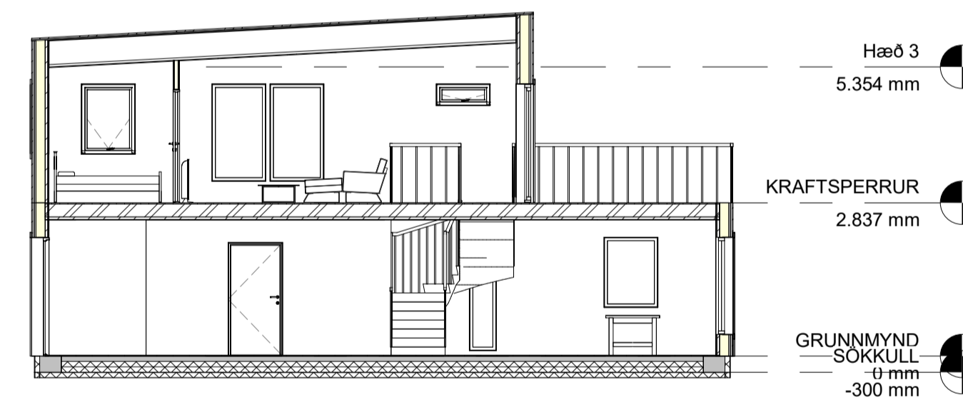
7 LANGSNID 1:100
