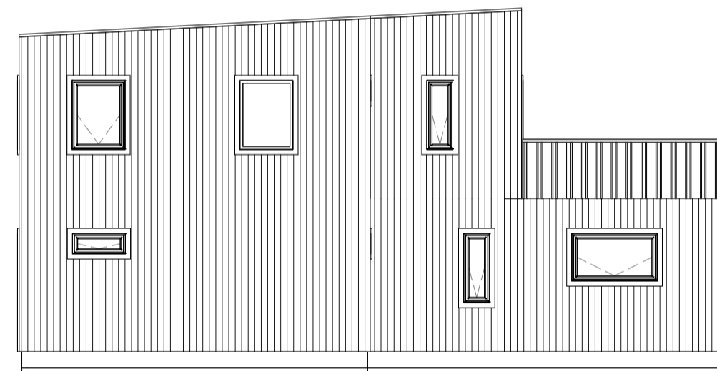
4 ÚTLIT 1 1:100
