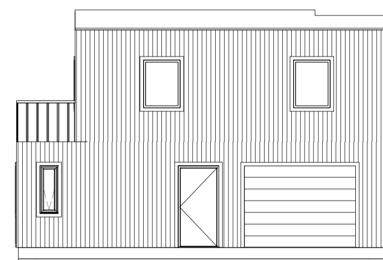
3 ÚTLIT 2 1:100
