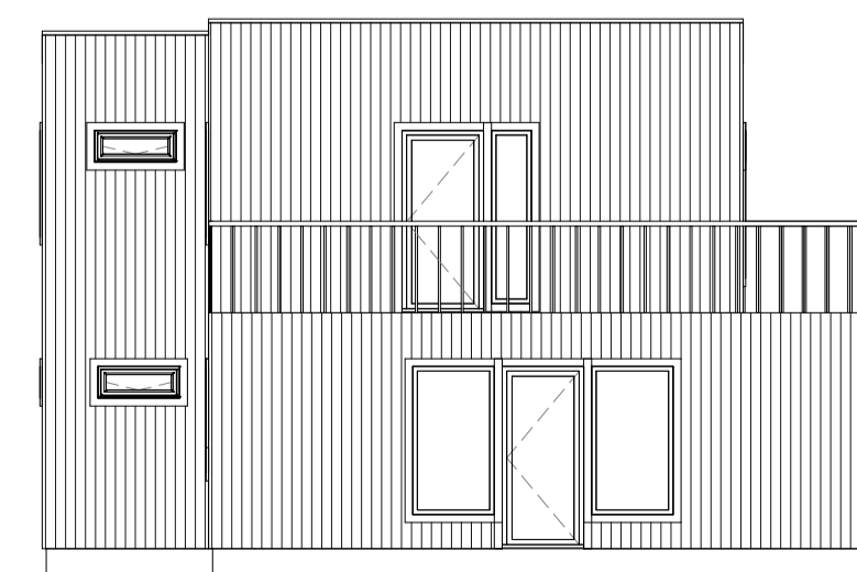
6 ÚTLIT 4 1:100
